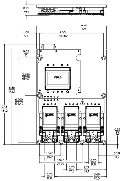
Configuration MVC-E / MVX-E LugMates
